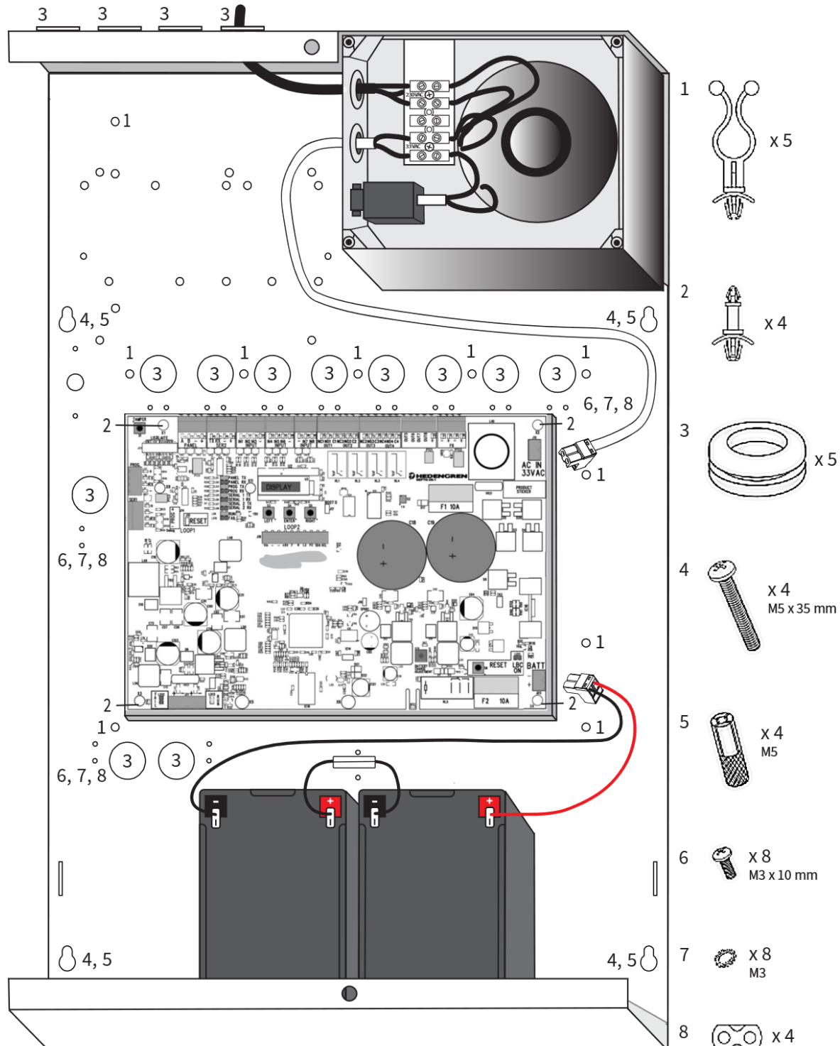
Figur 3 Tillbehör för installation
