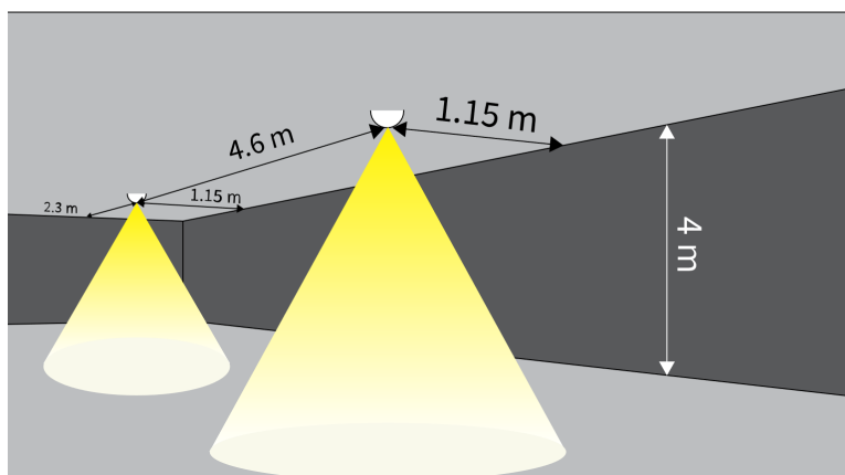
Figur 32 N68-C (5 lx, Centreline), takhöjd 4 m
