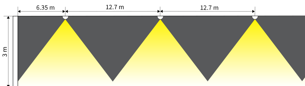
Figur 23 N68-C (1 lx, Centreline), takhöjd 3 m
