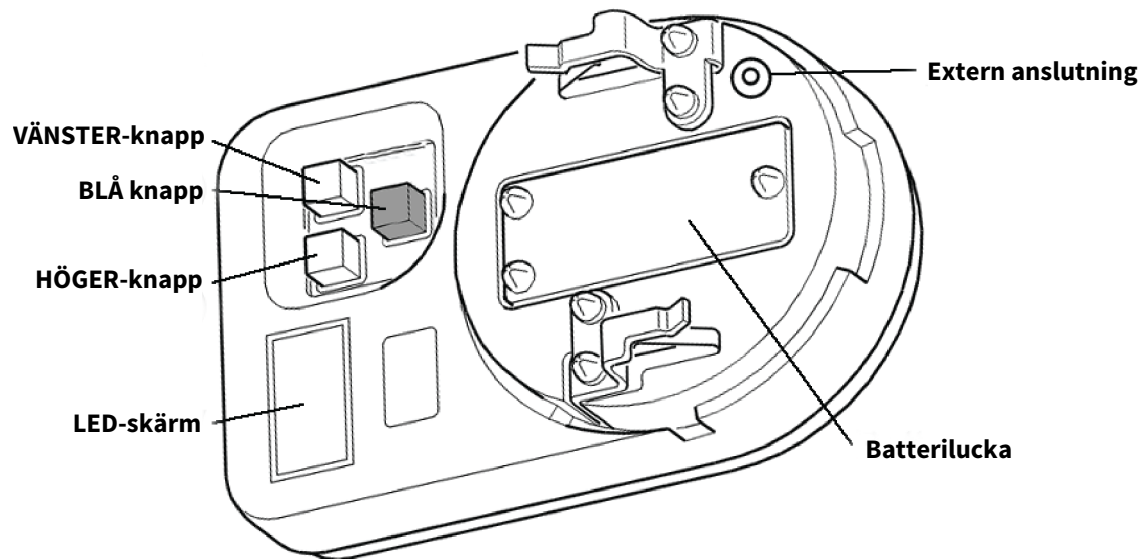
Figur 16 TCH-B200 Programmerare
