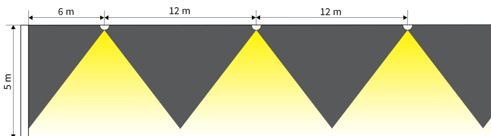
Figur 24 N68-C (1 lx, Centreline), takhöjd 5 m
