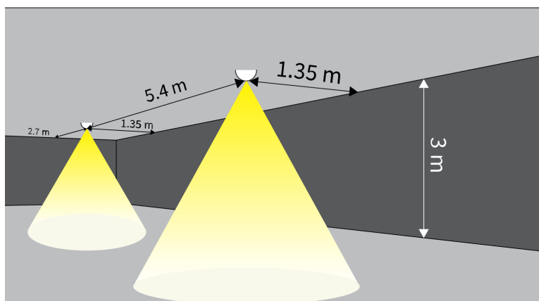
Figur 31 N68-C (5 lx, Centreline), takhöjd 3 m
